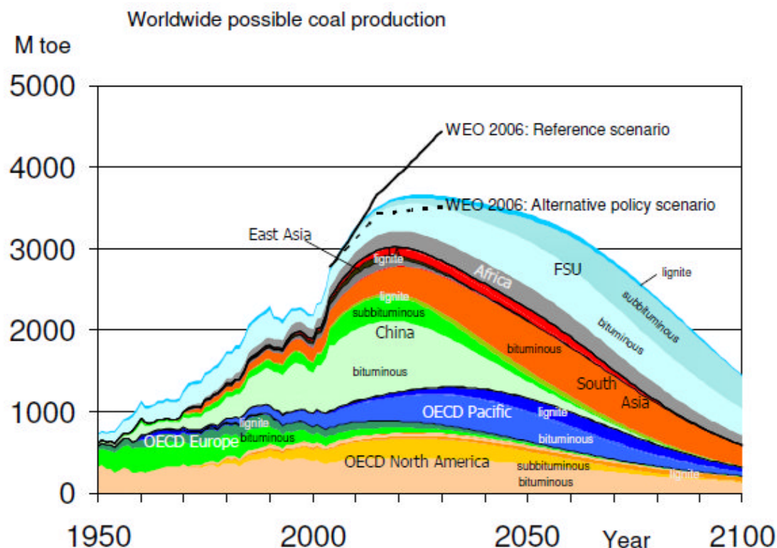
Figura 3. Evolución pasada y posible extracción futura mundial del carbón Fuente: Zittel y Schindler (2007) y Heinberg (2009).
