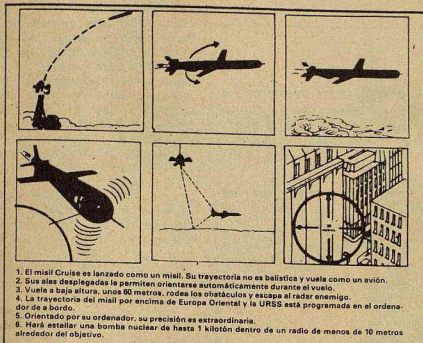
1. El misil Cruise se lanza como un misil. Su trayectoria no es balística y vuela como un avión. 2. Sus alas desplegadas le permiten orientarse automáticamente durante el vuelo. 3. Vuela a baja altura, unos 80 metros, rodea los obstáculos y escapa al radar enemigo. 4. La trayectoria del misil por encima de Europa Oriental y la URSS está programada en el ordenador de a bordo. 5. Orientado por su ordenador, su precisión es extraordinaria. 6. Hará estallar una bomba nuclear de hasta 1 kilotón dentro de un radio de menos de 10 metros alrededor del objetivo.
