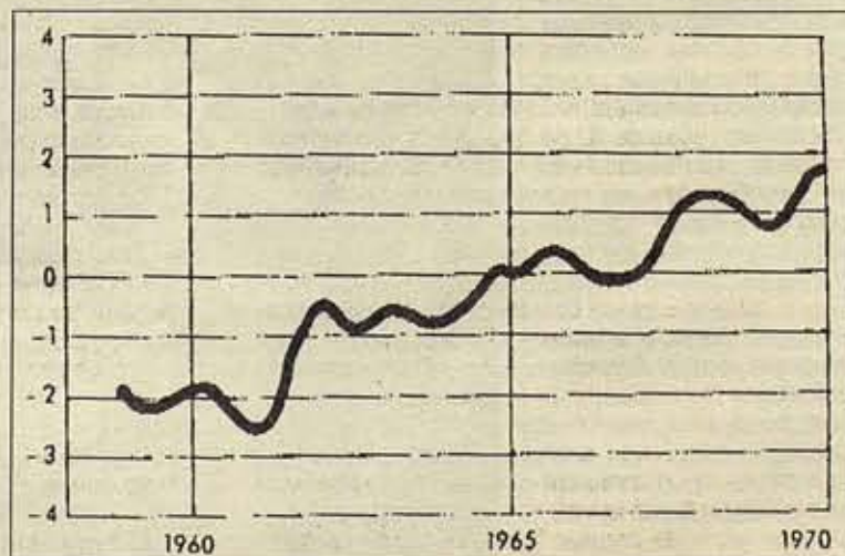
Desviaciones porcentuales sobre la media total de ozono
