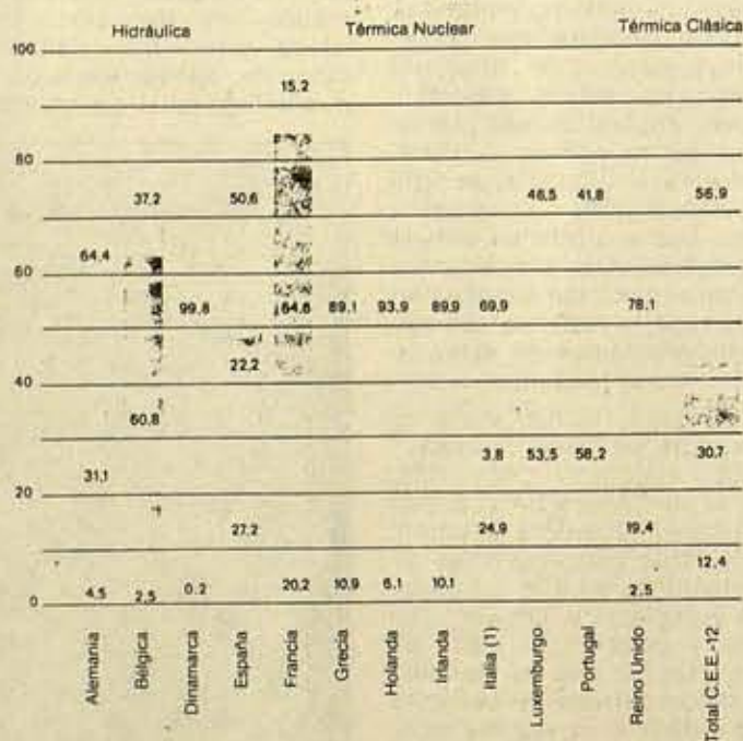
Participación de la energía nuclear en la producción total de energía. De abajo a arriba las cifras corresponden a energía térmica, nuclear e hidráulica.
